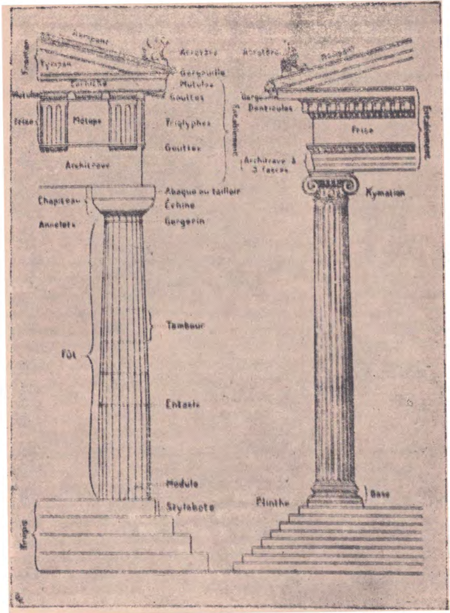
Çizim : 1 Yunan mabediin oluşturan ana unsurlar:
