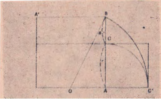
Çizim : 2 Euclide Okulunda Altın kesim'in çizimi
